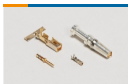
连接器端子(94)
