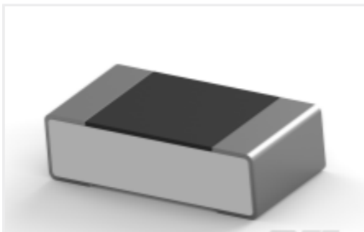
TE 产品编号 4-2176370-4 RQ 0603 1K21 0.1% 10PPM 5K RL
