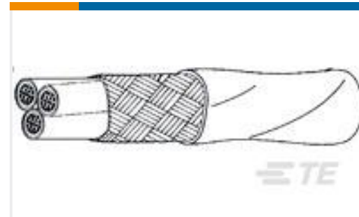
TE 产品编号3822713001 44A1131-20-0/1/9-9
