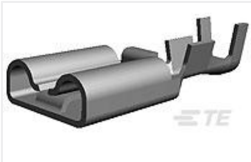
TE 产品编号175020-1 250 PL EX REC. 22-18AWG PTBR
