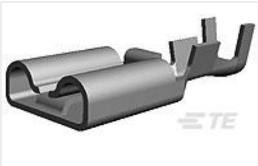
TE 产品编号175022-1 250 PL EX REC. 18-14AWG PTBR
