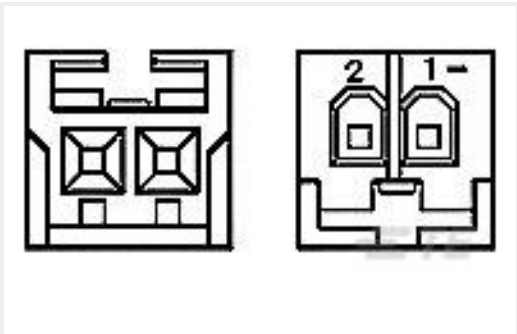
TE 产品编号172486-3 3P REC HSG CRIMP EI SER
