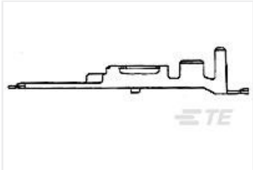
TE 产品编号172779-1 MIC MARK-2 TAB CONTACT
