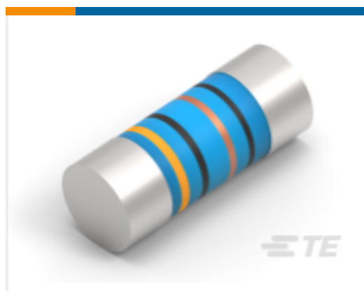
TE 产品编号2-2176316-1 MELF SMA_A 4K7 0.1% 15PPM 0207 1W
