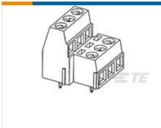
TE 产品编号796692-3 TERMI-BLOK PCB MOUNT 1&2 3P.5
