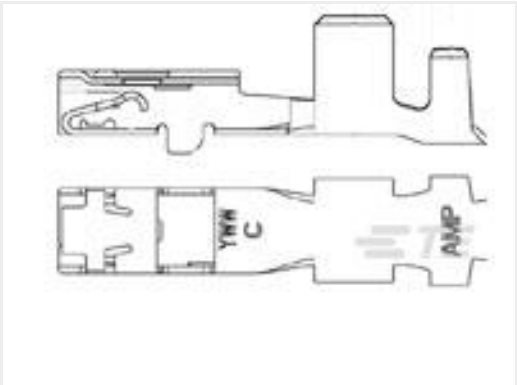
TE 产品编号1326030-4 2.8MM RECP,UNSEAL,10-12AWG
