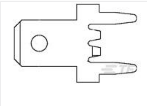
TE 产品编号63982-1 187 FASTON TAB TPBR
