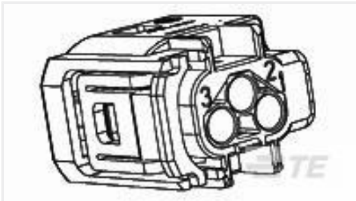
TE 产品编号1376235-1 MQS SOCKET HSG 3P ASSY
