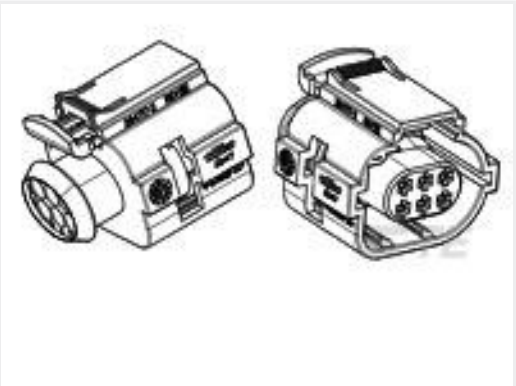
TE 产品编号284716-4 6 P. REC CONN X UEGO CONN
