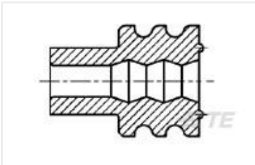
TE 产品编号963292-1 WIRE SEALING 2,2
