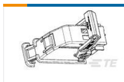
TE 产品编号284360-1 18 POS. FRAME ASSY FOR MQS CON
