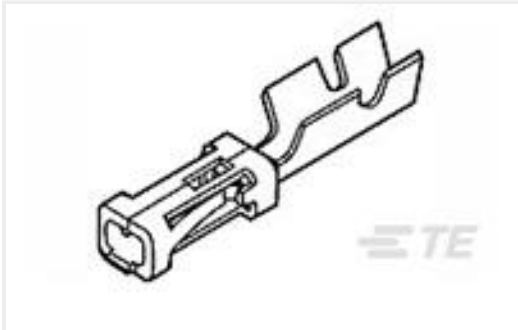
TE 产品编号86016-5 MOD IV RECP LP
