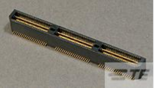
TE 产品编号 1-1658464-3 MSB0.80PL8ASY84DP,-,30,VCTY
