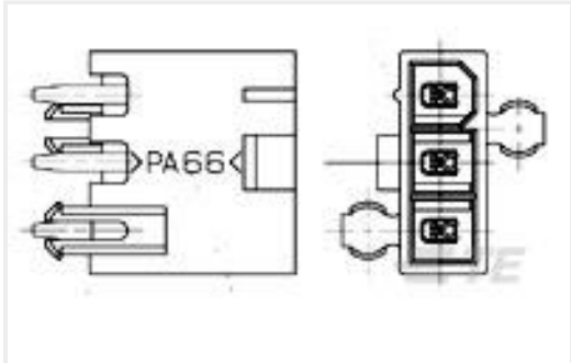
TE 产品编号2029056-3 3P VAL-U-LOK SR HDR SN V0 W/DH
