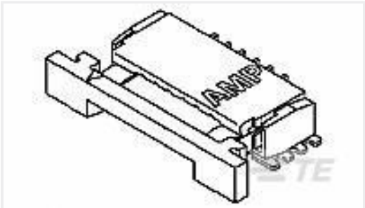
TE 产品编号1-84952-0 1MM FPC HORZ.BTTM CONT.ASS.10P
