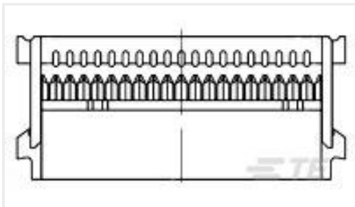
TE 产品编号1658526-5 609-1041LF FEM SOCKT,LEAD FREE
