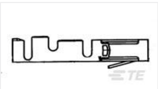
TE 产品编号280708-2 MOD 2 CONTACT
