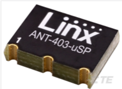
TE 产品编号ANT-403-USP-T Antenna uSP PCB RPC 403MHz SMT T&R
