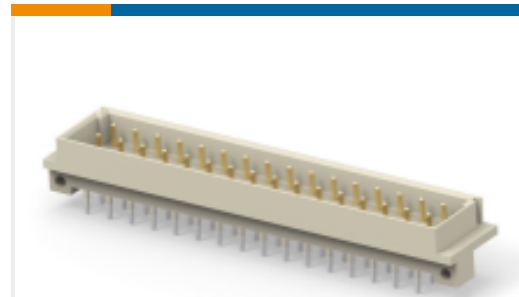
TE 产品编号364891-E STVE 48 M ACE GGG 4-00 GA16 3,8 * 247 E0
