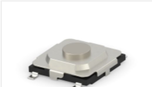
TE 产品编号2337237-1 TACT MINI GW 5.2X5.2X1.5 70GF
