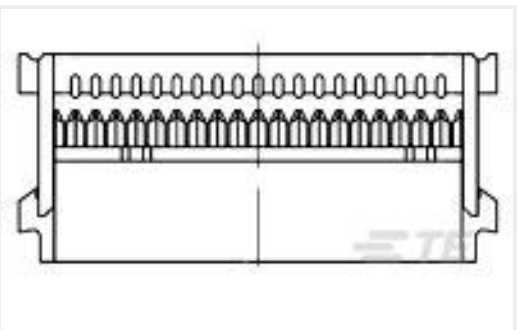
TE 产品编号2-1658526-9 609-1630LF=FSKT IDC S 16 30AU
