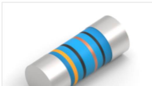
TE 产品编号7-2176316-2 MELF SMA_A 68K 1% 50PPM 0207 1W
