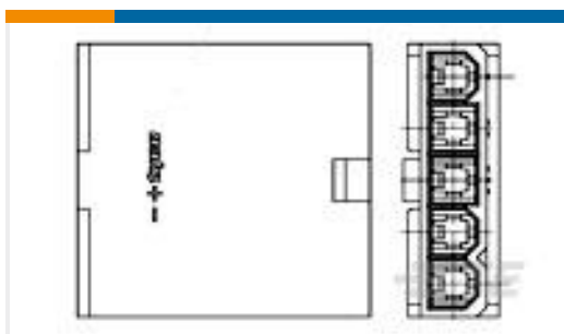
TE 产品编号1586024-5 5P S/R FH PLUG VAL-U-LOK V2
