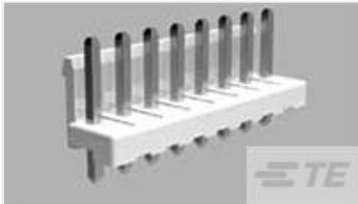
TE 产品编号1-1123723-2 3.96 EP HDR ASSY 2P(NATURAL)
