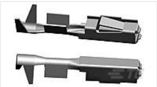
TE 产品编号2141824-1 MQS0,63 Sn rec LL unseal. 0,13-0,17
