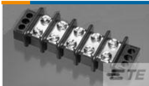
TE 产品编号 1-1546310-8 18P.563" DR BARRIER STRIP
