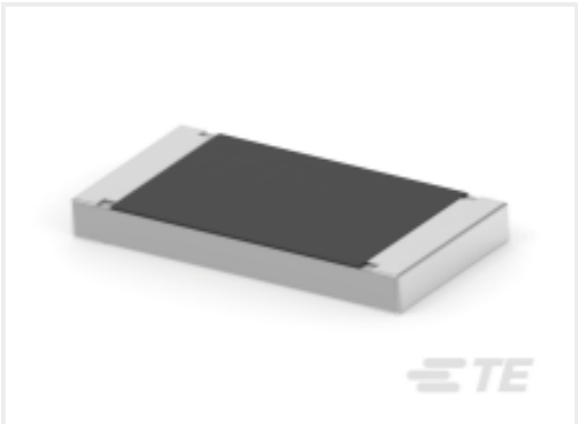
TE 产品编号1-2176350-3 CRGCQ 2512 100R 5%
