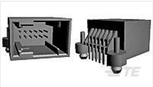
TE 产品编号185740-3 12pos MQS .63 header 90deg
