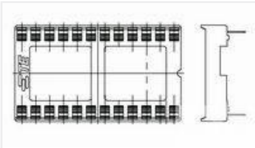
TE 产品编号1-2199299-5 40P,DIP SKT,600 CL,LDR,PB FREE
