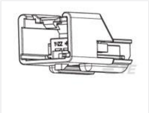
TE 产品编号6-1419166-1 1X4MALE IL ASSY "A"
