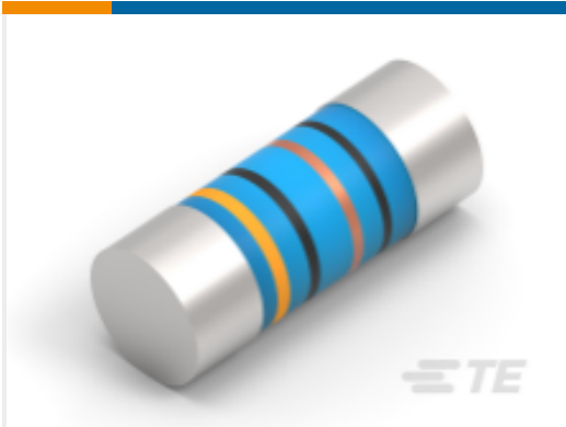
TE 产品编号1-2176316-5 MELF SMA_A 1K5 0.1% 15PPM 0207 1W
