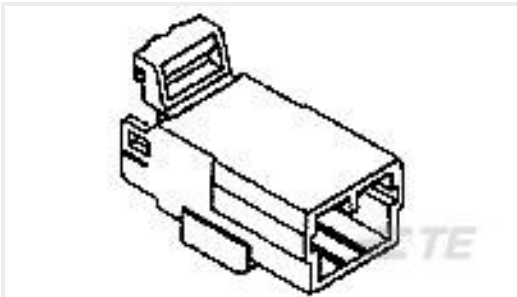
TE 产品编号1-174928-1 070 MLC W-W CAP HSG 3P F/A
