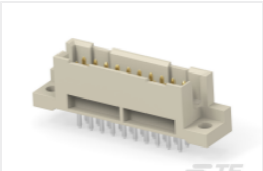
TE 产品编号374932-E STVQ/3 20 MI AB VV 4-00 GA06 4,0 * 247 E
