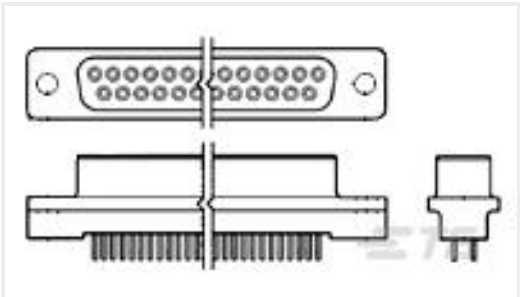
TE 产品编号5745058-3 HD-20 RCPT 25P VERT THD INS
