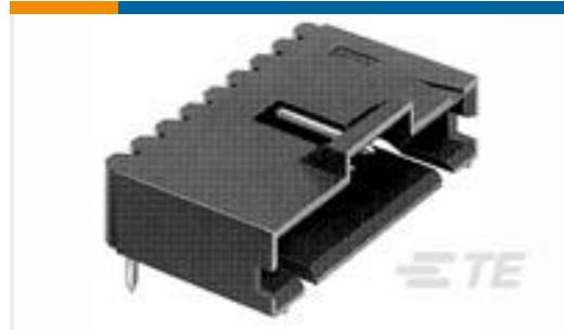
TE 产品编号 7-104935-3 24 MTE HDR SRRA LTCH.100CL LF
