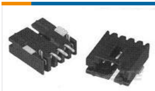
TE 产品编号 1-147278-5 16 MTE HDR SRRA SFMNT .100CL
