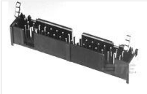
TE 产品编号104128-4 020 LOPRO HDR SP 30DP LATCH
