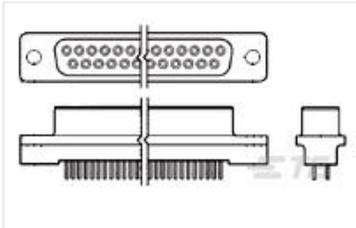
TE 产品编号5745059-4 HD-20 RCPT 37P VERT THD INS
