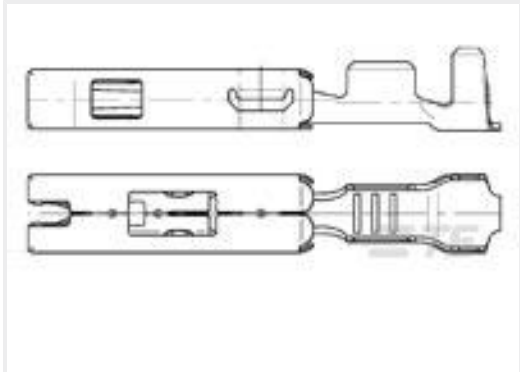
TE 产品编号929027-1 1.5MM SFC
