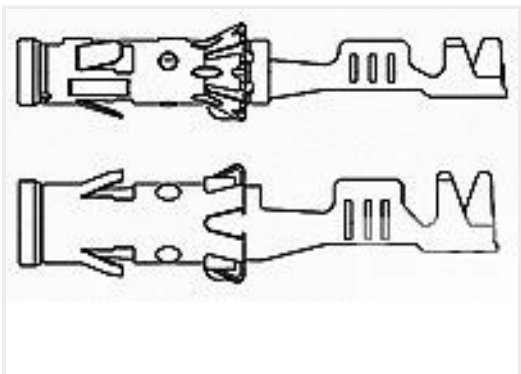
TE 产品编号962952-2 4MM BUCHS-KONTAKT
