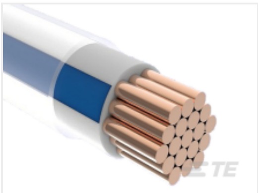
TE 产品编号3289243001 ACW0219-1.00-62(NS)
