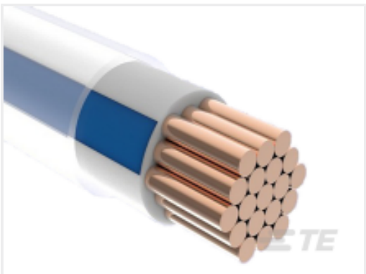
TE 产品编号4691263001 ACW0219-1.00-1(NS)
