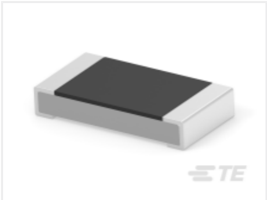
TE 产品编号4-2176392-5 RQ 1206 383K 0.1% 10PPM 5K RL
