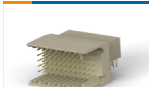
TE 产品编号106014-1 硬制背板公连接器：直角，共面， 2mm
