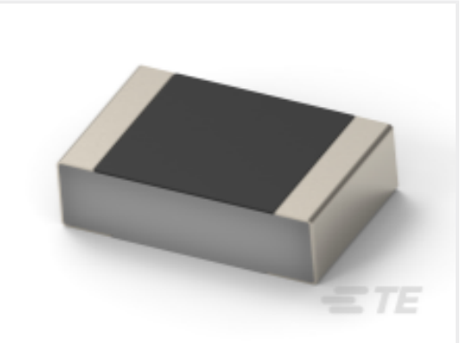
TE 产品编号9-2176453-2 CPF 0201 51K1 0.1% 25ppm 1K RL
