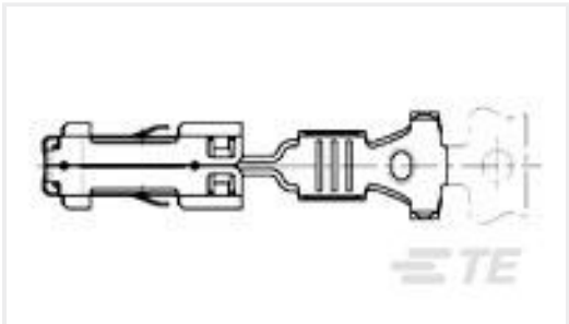
TE 产品编号1703034-1 SENSOR CONTACT 2,8
