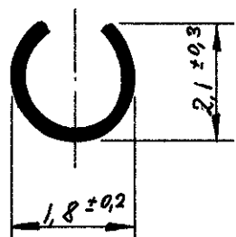
DRAHTPRESSHÜLSE
