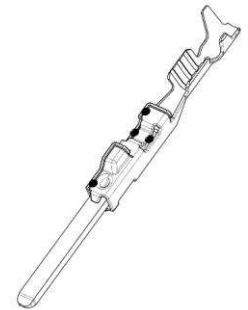
Fig. / Abb. 9: Wire and Insulation Crimp Dimensions / Draht- und Iso-Crimpmaße MCON 1.2 CB TAB
