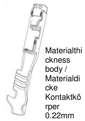
Fig. / Abb. 6: Wire and Insulation Crimp Dimensions / Draht- und Iso-Crimpmaße MCON 1.2 CB
