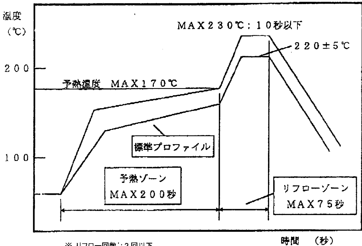
Fig.5 I.R.リフロー温度プロファイル
